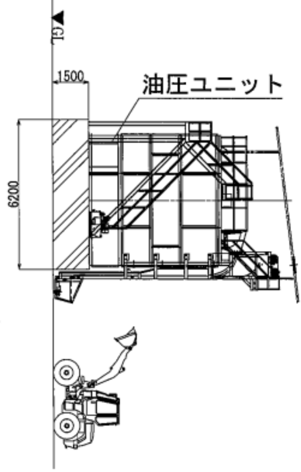
コンポS-90ET×2台 レイアウト参考図面 基礎1500mm
